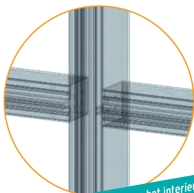
Koppeling van stijlen en dorpels
